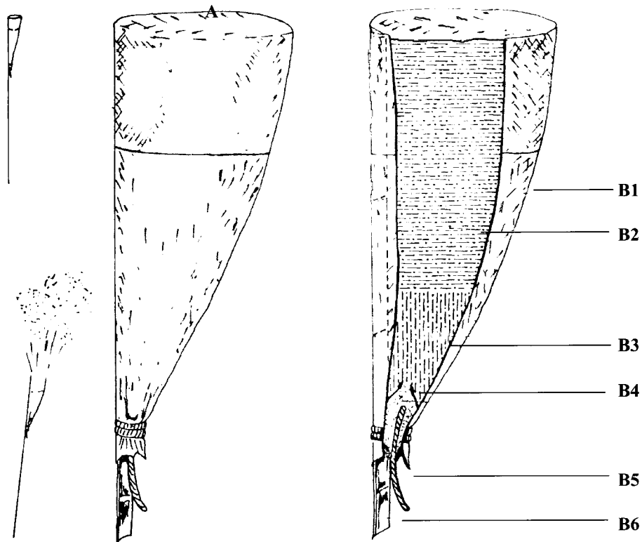
Cohete de flores A: Producto terminado B1: Cartucho de cartulina. B2: Papel de seda picado B3: Papel periódico. B4: Pólvora B5: Mecha. B6: Carrizo.
