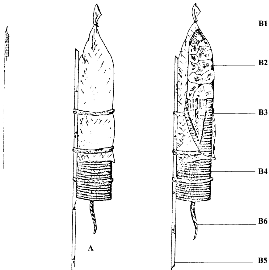
Cohete de luz A: Producto terminado B1: Papel periódico B2: Bombas de colores B3: Pólvora impulsora B4: Cabuya encerada B5: Carrizo B6: Mecha
