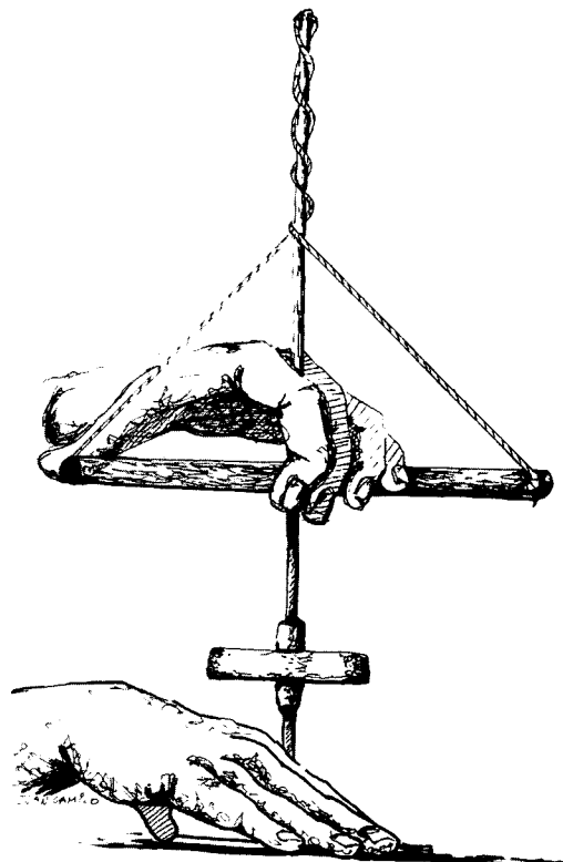
Taladro de piola
